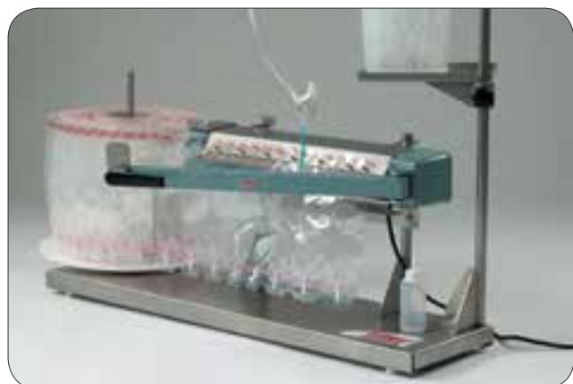
Ref. 022267 Envasadora manual GTB 250 Máquina envasadora y selladora manual. El flujo del semen se controla manualmente mediante un clamp. La velocidad de llenado es de 250 bolsas GTB por hora.
